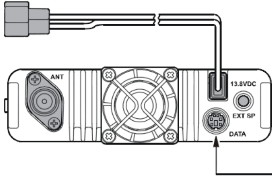
Схема подключения оборудования для скорости 9600 бит/с
